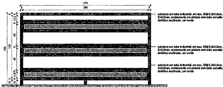
4 VISTA POSTERIOR - PRATELEIRA HORTIFRUTI 1 : 20
