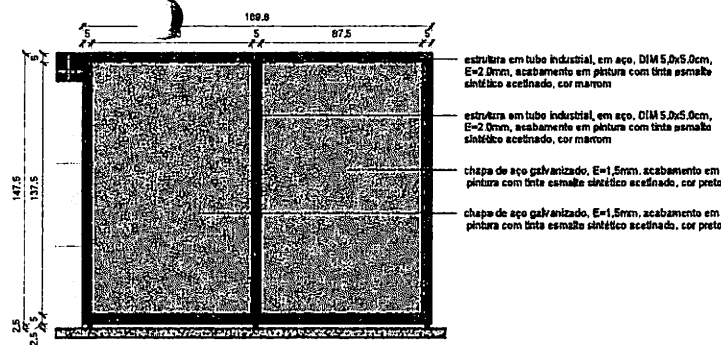
2 VISTA FRONTAL - DIVISÓRIA CAFÉ / LANCHE E CHURRASQUINHO
