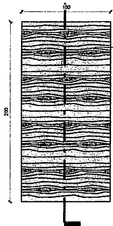
1 PLANTA BAIXA - MESA HORTIFRUTI 1:20
