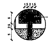
6 DETALHAMENTO - DIVISÓRIA CHEIRO VERDE / TEMPERO SECO 1:5
