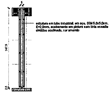
3 VISTA LATERAL - DIVISÓRIA BANANA E FARINHA 1:20
