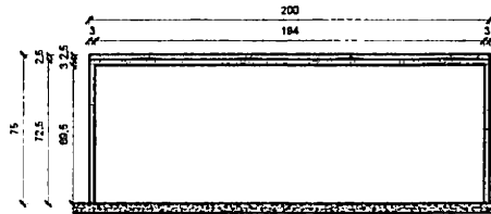
3 VISTA LATERAL - MESA HORTIFRUTI 1:20
