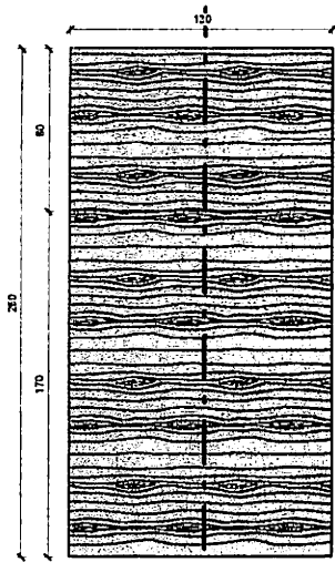
1 PLANTA BAIXA - MESA BANANA 1:20
