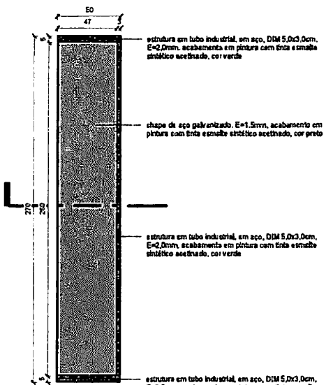
1 PLANTA BAIXA - PRATELEIRA HORTIFRUTI 1 : 20
