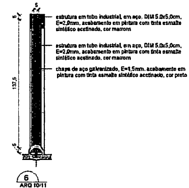
5 CORTE - DIVISÓRIA CAFÉ / LANCHE E CHURRASQUINHO
