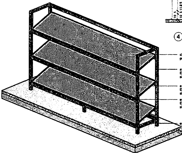
7 VISTA VOLUMÉTRICA - PRATELEIRA HORTIFRUTI
