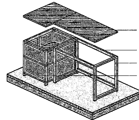
9 WV - MESA CHEIRO VERDE / TEMPERO SECO EXPLODIDO
