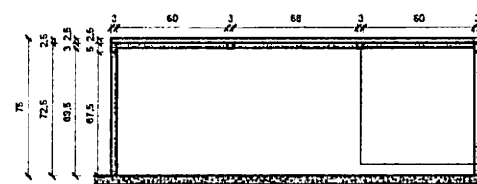
4 CORTE - MESA HORTIFRUTI 1:20
