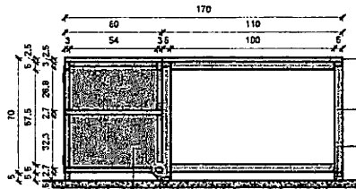
1 PLANTA BAIXA - MESA CHEIRO VERDE / TEMPERO SECO 1:20
