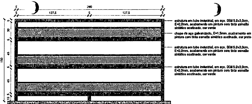
2 VISTA FRONTAL - PRATELEIRA HORTIFRUTI 1 : 20
