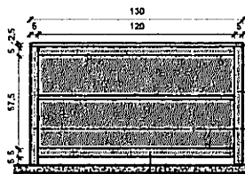
2 VISTA FRONTAL - MESA VARIEADES 1 : 20
