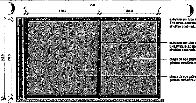
2 VISTA FRONTAL - DIVISÓRIA CHEIRO VERDE / TEMPERO SECO 1:20
