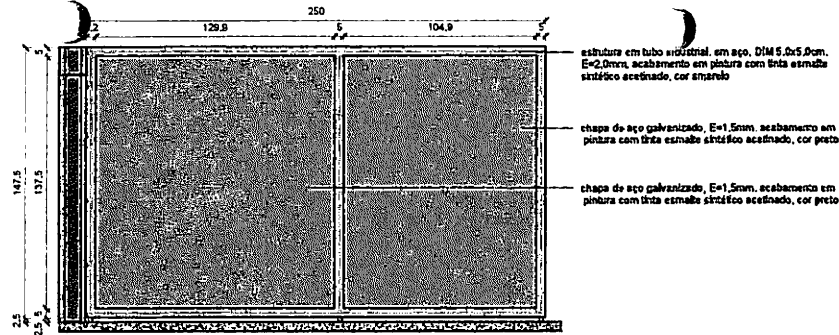
2 VISTA FRONTAL - DIVISÓRIA BANANA E FARINHA 1:20
