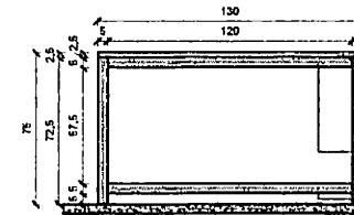
4 VISTA LATERAL DIREITA - MESA BANANA 1:20
