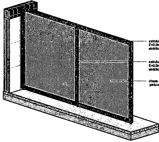
6 VISTA VOLUMÉTRICA - DIVISÓRIA HORTIFRUTI
