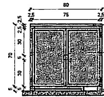
4 VLE - MESA CHEIRO VERDE / TEMPERO SECO 1:20
