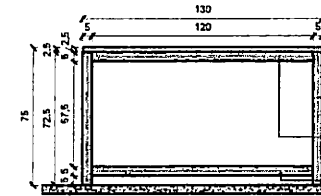
3 VISTA LATERAL ESQUERDA - MESA BANANA 1:20
