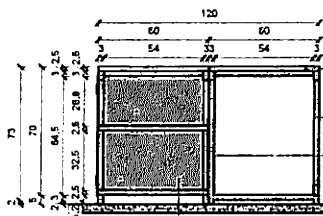
4 VISTA LATERAL ESQUERDA - MESA VARIEADES 1 : 20
