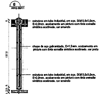
5 CORTE - DIVISÓRIA BANANA E FARINHA 1:20
