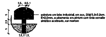
6 DETALHAMENTO - DIVISÓRIA CAFÉ / LANCHE E CHURRASQUINHO
