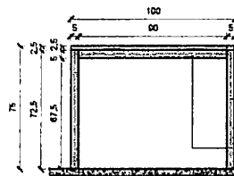
2 VISTA FRONTAL - MESA HORTIFRUTI 1:20
