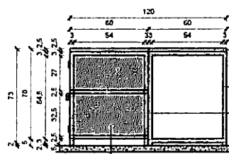
3 VISTA LATERAL DIREITA - MESA VARIEADES 1 : 20
