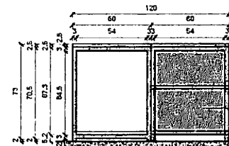
3 VISTA LATERAL DIREITA - MESA VARIEADES 1 : 20
