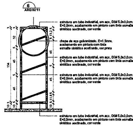
5 CORTE - PRATELEIRA HORTIFRUTI 1 : 20
