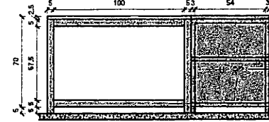
5 VISTA POSTERIOR - MESA CHEIRO VERDE / TEMPERO SECO 1:20
