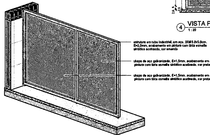
7 VISTA VOLUMÉTRICA - DIVISÓRIA BANANA E FARINHA
