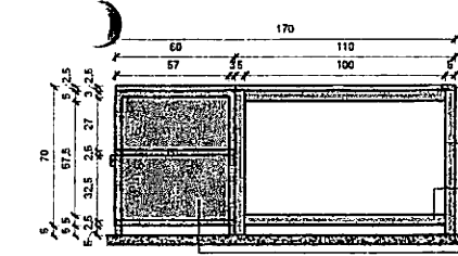
2 VISTA FRONTAL - MESA CHEIRO VERDE / TEMPERO SECO 1:20
