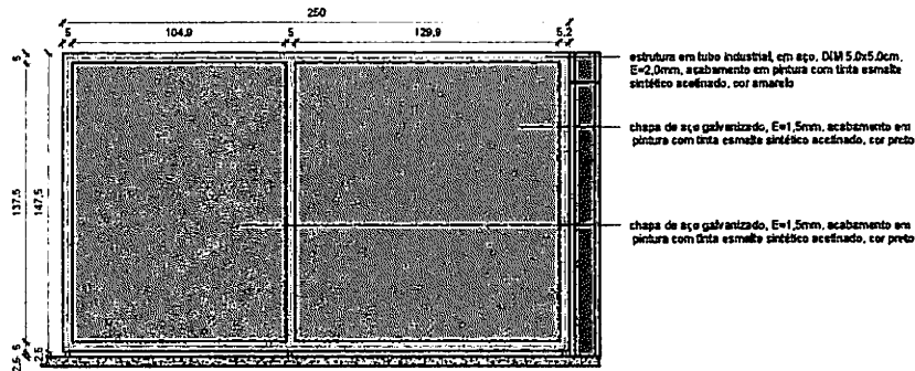
4 VISTA POSTERIOR - DIVISÓRIA BANANA E FARINHA 1:20
