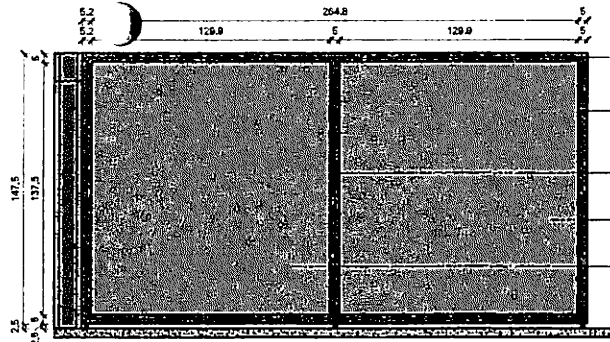
2 VISTA FRONTAL - DIVISÓRIA HORTIFRUTI 1:20
