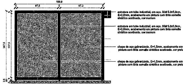
4 VISTA POSTERIOR - DIVISÓRIA CAFÉ / LANCHE E CHURRASQUINHO
