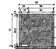
3 VLD - MESA CHEIRO VERDE / TEMPERO SECO 1:20
