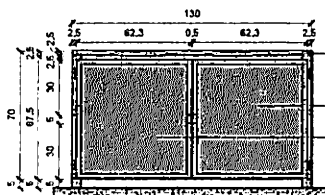
3 VISTA POSTERIOR - MESA VARIEADES 1 : 20
