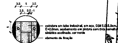
6 DETALHAMENTO - DIVISÓRIA BANANA E FARINHA 1:5
