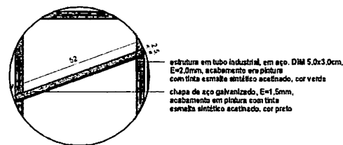
6 DETALHAMENTO - PRATELEIRA HORTIFRUTI 1 : 10
